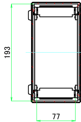
A-A ( 1 : 4.5 )
